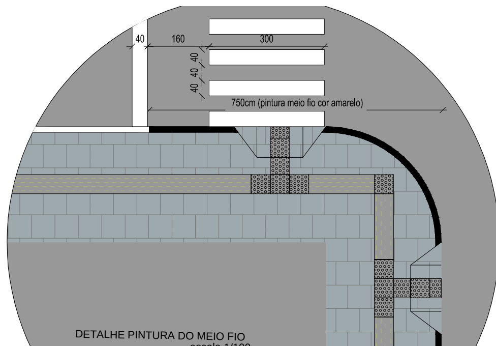
DETALHE ESQUINA E FAIXA DE PEDESTRE ESCALA 1/100
