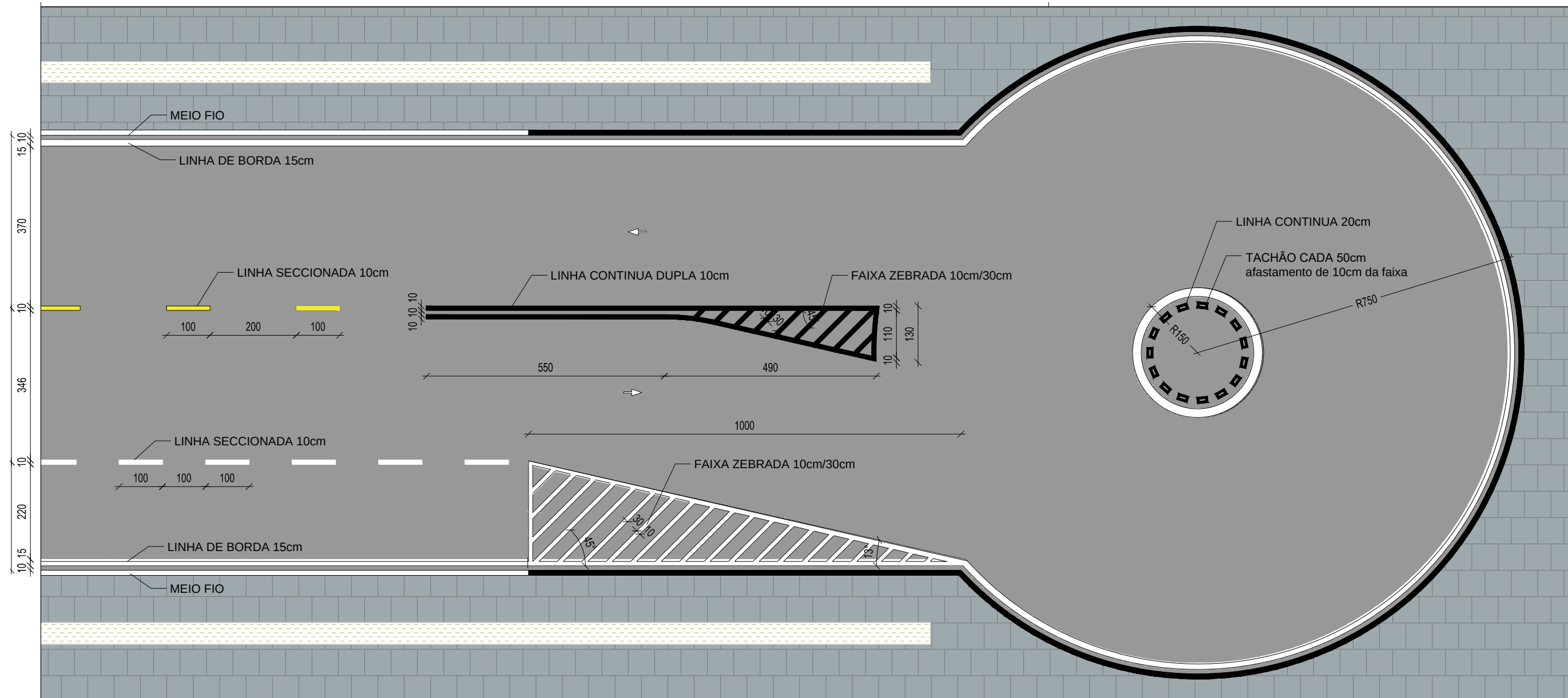
DETALHE SINALIZAÇÃO HORIZONTAL E CUL-DE-SAC ESCALA 1/100
