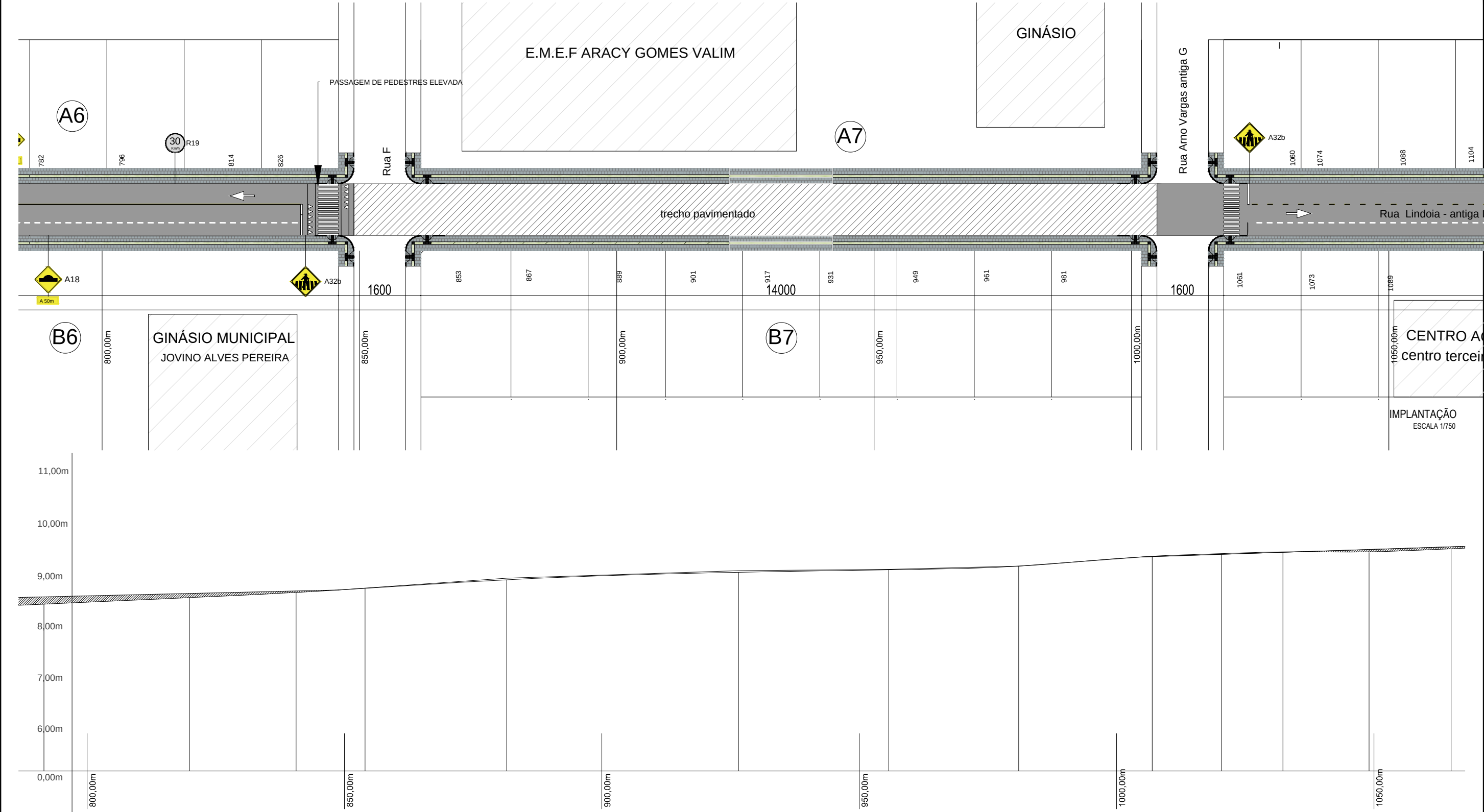
CORTE LONGITUDINAL ESCALA 1/750
