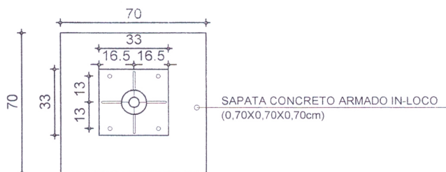
BASE DO POSTE METÁLICO (0,33X0,33cm)
