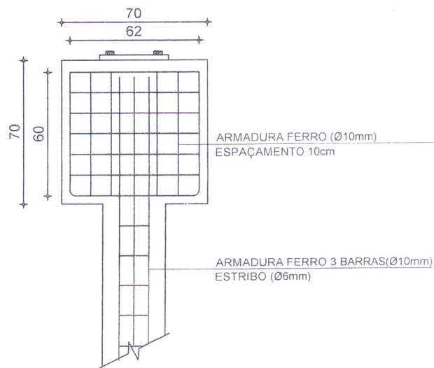
CORTE ARMADURA DUPLA FERRO SAPATA
