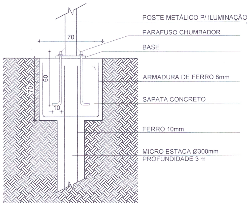
DETALHE BASE P/ POSTE METÁLICO P/ ILUMINAÇÃO ESCALA: 1/25
