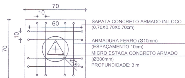
PLANTA ARMADURA DUPLA FERRO SAPATA
